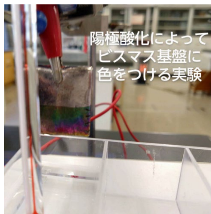
↑ ビスマスの電気分解による 着色と脱色の様子
